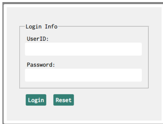
登陆界面
