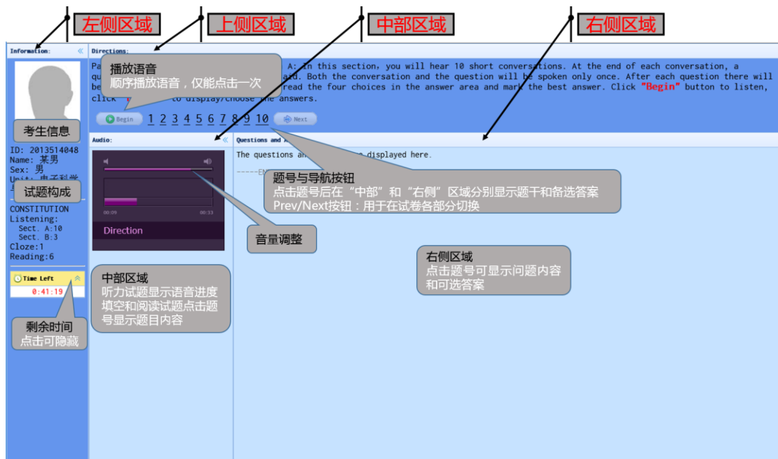
系统主界面
